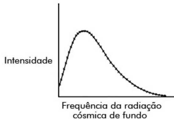
Figura 9.1. A linha sólida representa a previsão feita pela teoria do Big Bang, segundo a qual a radiação cósmica de fundo deveria se assemelhar à radiação do corpo negro na região das micro-ondas. Os x representam os dados reais coletados pelo satélite COBE, fornecendo-nos uma das mais convincentes provas da teoria do Big Bang.
