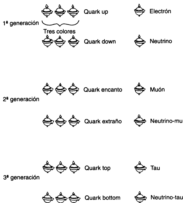
Figura 5.4. En el Modelo Estándar, la primera generación de partículas consta de los quarks up y down (en tres colores, con sus antipartículas asociadas) y el electrón y el neutrino. La característica embarazosa del Modelo Estándar es que existen tres generaciones de tales partículas, siendo cada generación casi una copia exacta de la generación anterior. Resulta difícil creer que la naturaleza fuera tan redundante como para crear, en un nivel fundamental, tres copias idénticas de partículas.
