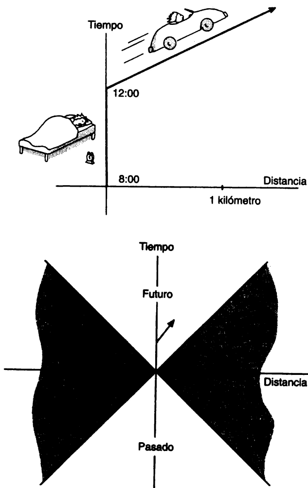
Figura 11.1. Nuestra línea de universo resume toda nuestra historia, desde el nacimiento a la muerte. Por ejemplo, si permanecemos en la cama desde las 8 hasta las 12, nuestra línea de universo es una línea vertical. Si vamos en automóvil al trabajo, entonces nuestra línea de universo se inclina. Cuanto más deprisa nos movemos, más se inclina nuestra línea de universo. Sin embargo, la velocidad más rápida a la que podemos viajar es la velocidad de la luz. Por consiguiente, una parte de este diagrama espacio-temporal está «prohibida»; es decir, tendríamos que ir a mayor velocidad que la luz para entrar en esta zona prohibida.
