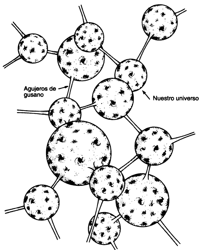
Figura 12.2. Nuestro universo puede ser uno entre un número infinito de universos paralelos, cada uno de los cuales está conectado a los demás por una serie infinita de agujeros de gusano. El viaje por estos agujeros de gusano es posible pero extremadamente improbable.
