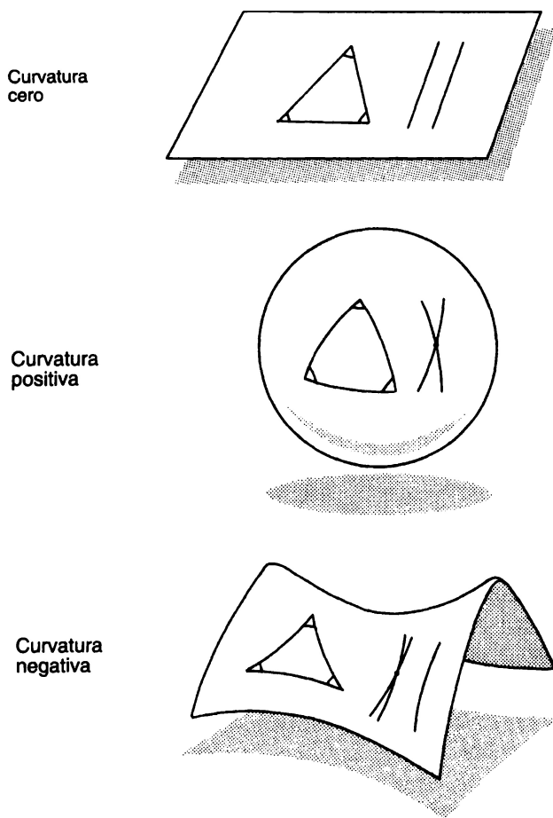
Figura 2.2. Un plano tiene curvatura cero. En la geometría euclidiana, los ángulos internos de un triángulo suman 180 grados, y las líneas paralelas nunca se cortan. En la geometría no euclidiana, una esfera tiene curvatura positiva. Los ángulos internos de un triángulo suman más de 180 grados y las líneas paralelas siempre se cortan. (Las líneas paralelas incluyen arcos cuyos centros coinciden con el centro de la esfera. Esto descarta las líneas de latitud constante.) Una silla de montar tiene curvatura negativa. Los ángulos internos suman menos de 180 grados. Existe un número infinito de líneas paralelas a una línea dada que pasan por un punto fijo.
