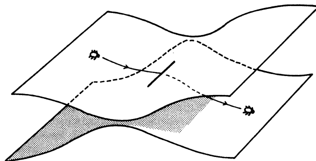
Figura 2.4. Un corte de Riemann, con dos hojas conectadas a lo largo de una línea. Si caminamos alrededor del corte, permanecemos dentro del mismo espacio. Pero si atravesamos el corte, pasamos de una hoja a la contigua. Ésta es una superficie múltiplemente conexa.
