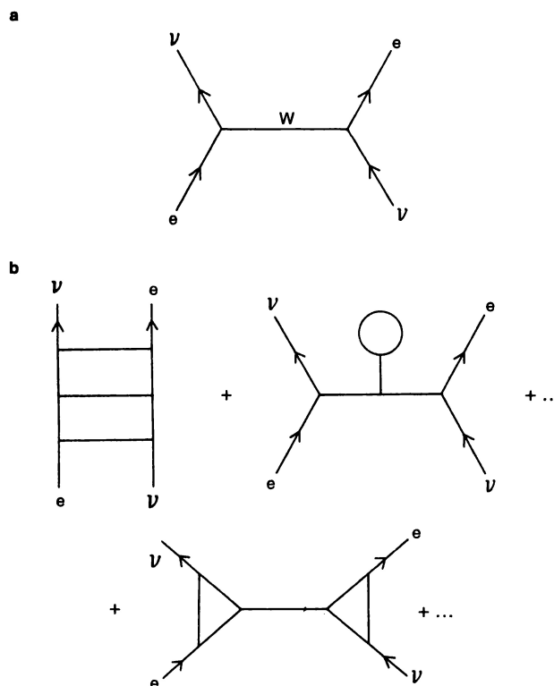
Figura 5.2. a) En teoría cuántica, cuando una partícula subatómica choca con otra, ambas intercambian paquetes de energía, o cuantos. Los electrones y los neutrinos interactúan intercambiando un cuanto de la fuerza débil, llamado partícula W. b) Para calcular la interacción completa de electrones y neutrinos, debemos sumar una serie infinita de grafos, llamados diagramas de Feynman, en los que los cuantos se intercambian de acuerdo
