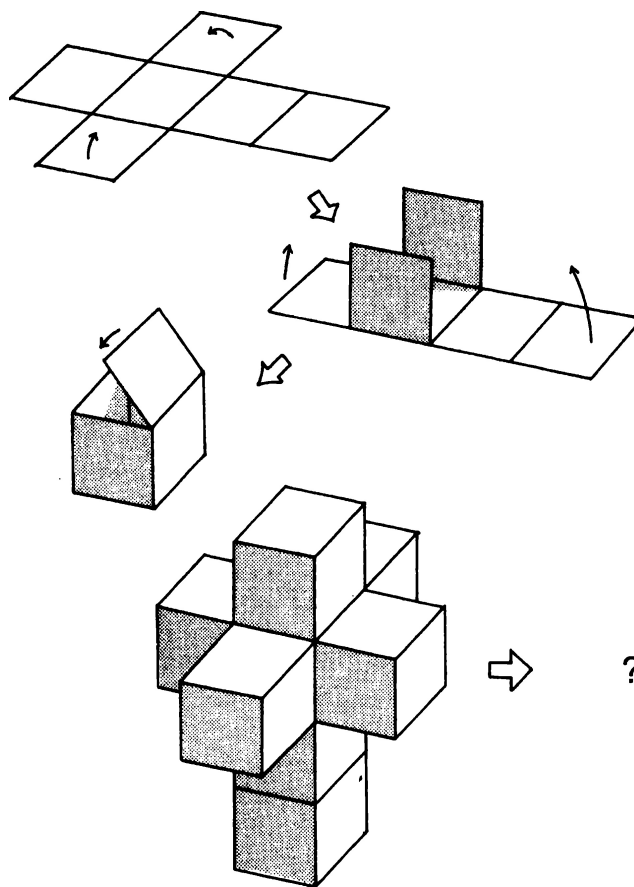
Figura 3.6. Los planilandeses no pueden visualizar un cubo, pero pueden hacerse una idea de un cubo tridimensional desplegándolo. Para un planilandés, un cubo desplegado se parece a una cruz que consiste en seis cuadrados. Análogamente, nosotros no podemos visualizar un hipercubo tetradimensional, pero si lo desplegamos, tenemos una serie de cubos dispuestos en un tesseract similar a una cruz. Aunque los cubos de un tesseract parecen inmóviles, una persona tetradimensional puede «doblar» los cubos en un hipercubo.
