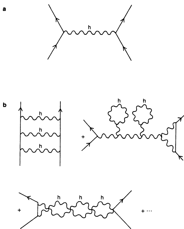
Figura 6.1. a) En teoría cuántica, un cuanto de la fuerza gravitatoria, señalado con h , se denomina gravitón, que se forma al romper la métrica de Riemann. En esta teoría, los objetos interactúan intercambiando este paquete de gravedad. De esta forma, hemos perdido completamente la bella imagen geométrica de Einstein. b) Por desgracia, todos los diagramas que contienen lazos cerrados son infinitos, lo que ha impedido una unificación de la gravedad con la teoría cuántica durante el último medio siglo. Una teoría cuántica de la gravedad que la una con las otras fuerzas es el Santo Grial de la física.
