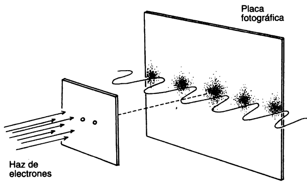
Figura 5.1. Se lanza un haz de electrones a través de dos pequeños agujeros tras los cuales hay una placa fotográfica expuesta. Esperamos ver dos manchas en la placa. En lugar de ello, encontramos una figura de interferencia ondulatoria. ¿Cómo puede ser? Según la teoría cuántica, el electrón es en realidad una partícula de tipo puntual y no puede atravesar ambos agujeros a la vez, pero la onda de Schrödinger asociada con cada electrón puede atravesar ambos agujeros e interferir consigo misma.
