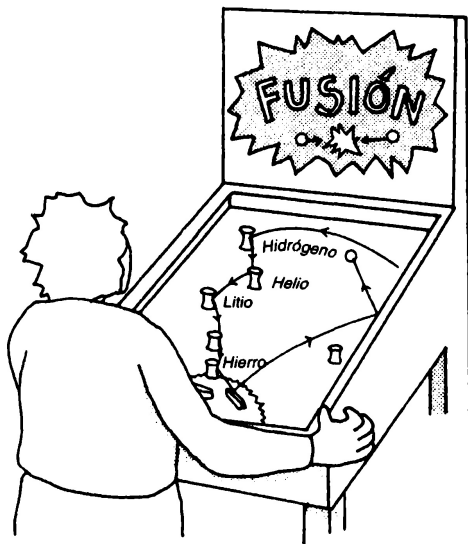
Figura 10.1. El «peso» promedio de cada protón de los elementos ligeros, tales como hidrógeno y helio, es relativamente grande. Por lo tanto, si fusionamos hidrógeno para formar helio dentro de una estrella, tenemos un exceso de masa, que se convierte en energía según la ecuación de Einstein E = mc^2 . Ésta es la energía que ilumina las estrellas. Pero a medida que las estrellas fusionan elementos cada vez más pesados, llegamos finalmente al hierro, y ya no podemos extraer más energía. Entonces la estrella colapsa, y el tremendo calor del colapso crea una supernova. Esta colosal explosión destruye la estrella y siembra el espacio interestelar, en el que se forman nuevas estrellas. Entonces vuelve a comenzar el proceso entero, como en un billar eléctrico.
