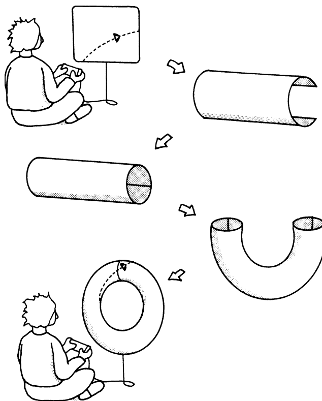
Figura 9.2. Si desaparece un cohete por el lado derecho de una pantalla de videojuegos, reemerge en el lado izquierdo. Si desaparece en la parte superior, reemerge en la parte inferior. Dobleemos ahora la pantalla de modo que empalmen los puntos idénticos. Primero empalmamos los puntos superiores y los inferiores curvando la pantalla. Luego empalmamos los puntos de la izquierda con los puntos de la derecha enrollando la pantalla como un tubo. De este modo, podemos mostrar que una pantalla de videojuegos tiene la topología de un toro.
